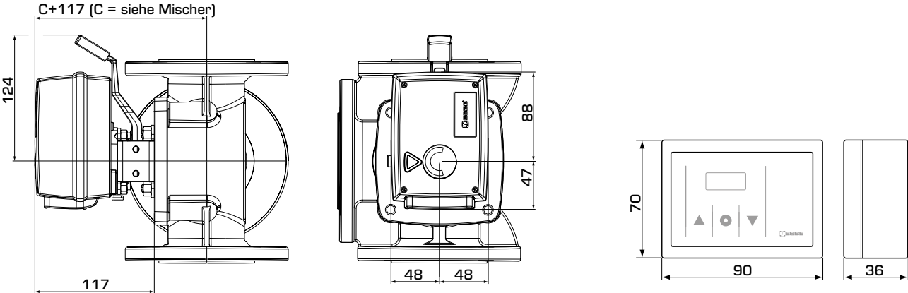
Einbauabmessungen für Kontroll- und Regeleinheit
