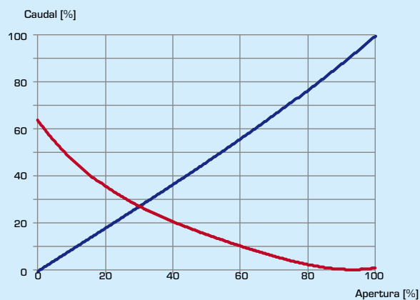
VLG132/VLG142, Kv 1,0, 1,6
