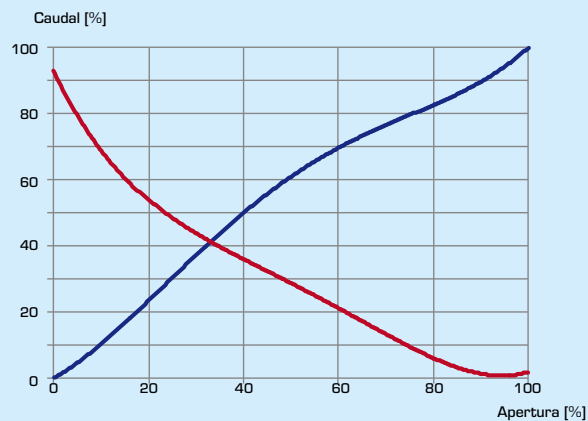
VLG132/VLG142, Kv 0,25, 0,4, 0,63
