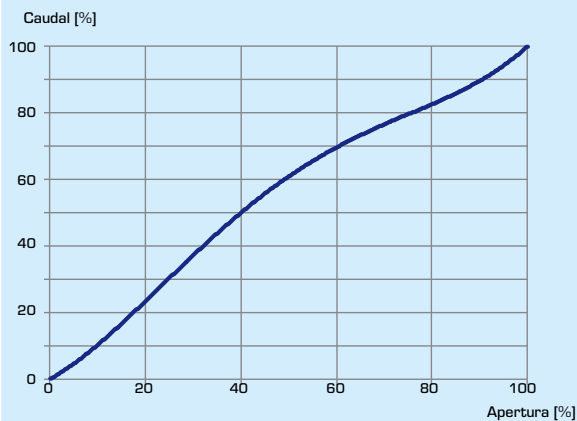
VLG122, Kv 0,25, 0,4, 0,63
