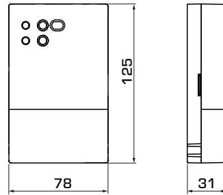
TWR911, ricevitore
