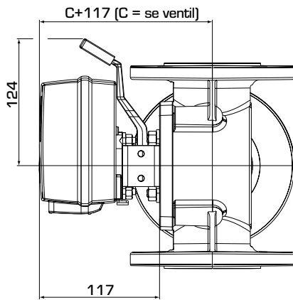
Installationsmått för reglering serie CRC120
