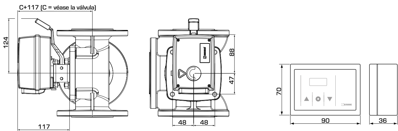
Dimensiones de instalación para el controlador serie CRA120
